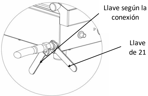
FIGURA 2 – CONEXIÓN
