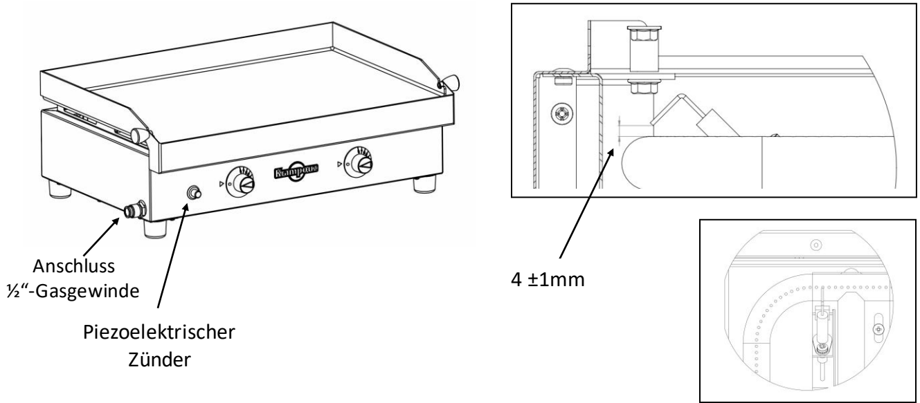
ABBILDUNG 2 – ANSCHLUSS
